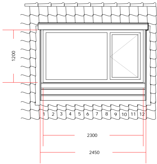
Dakkapel aanzicht schaal 1:50
