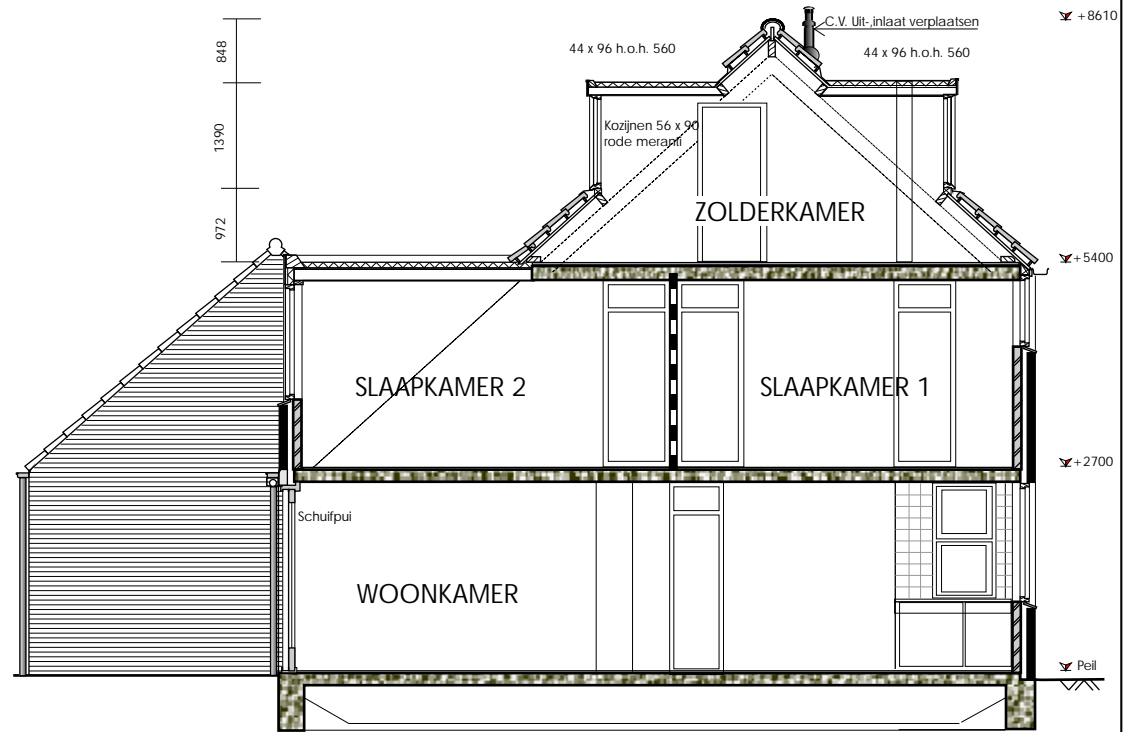
DOORSNEDE A-A
