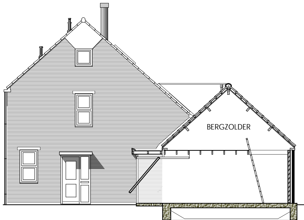
DOORSNEDE B-B
