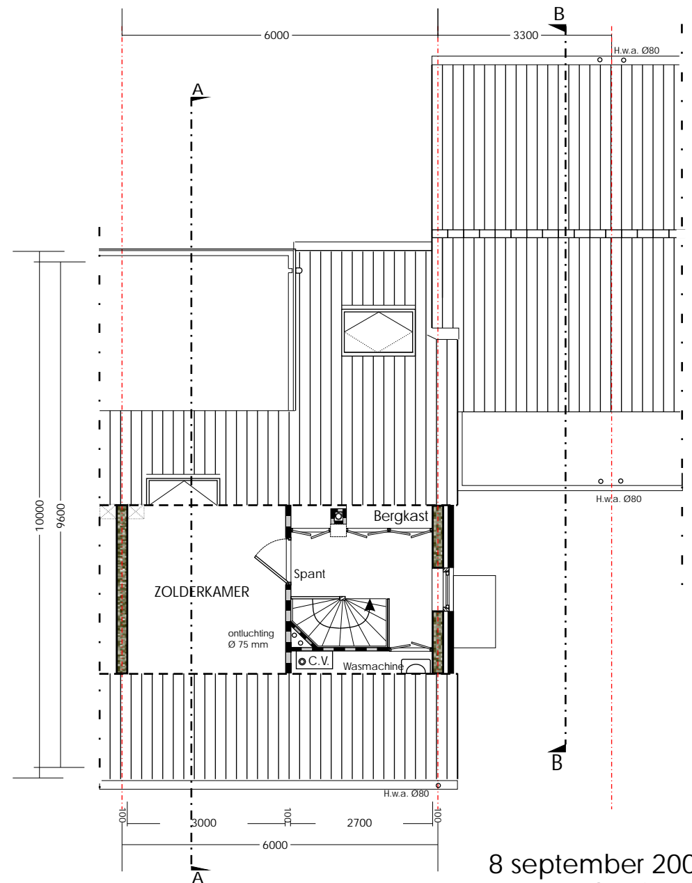
2e VERDIEPING
