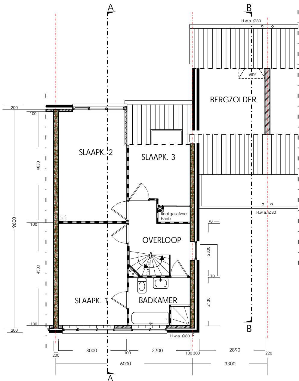
1e VERDIEPING
