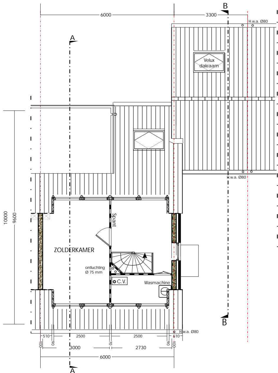
2e VERDIEPING
