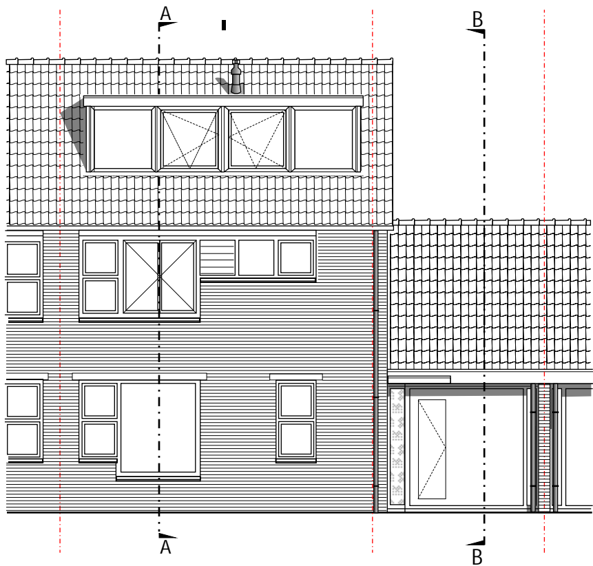
STRAATGEVEL
